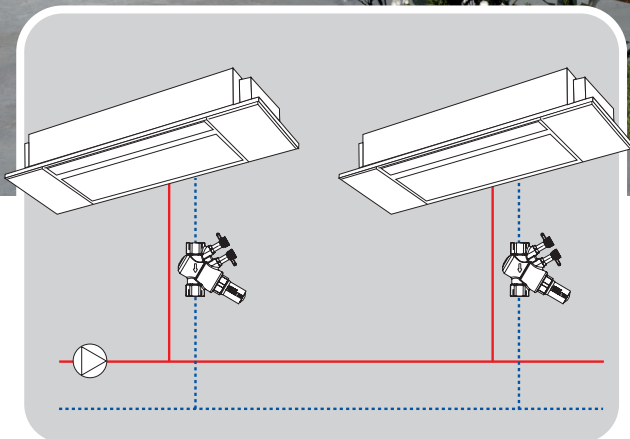
Fan Coil
